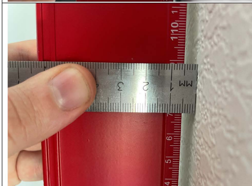
Фото №8. Измерение уровня стен в детской в квартире.
