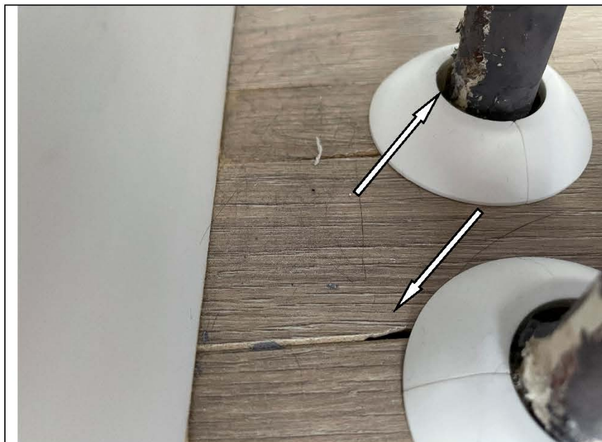
Фото №19. Заделка труб отопления в напольном покрытии в спальне.
