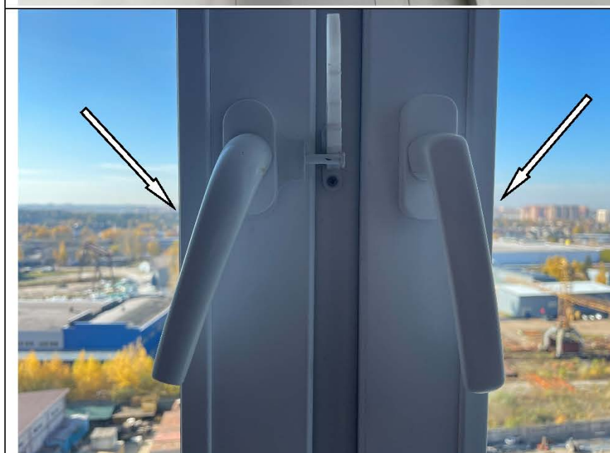
Фото №29. Фурнитура в спальне не отрегулирована.
