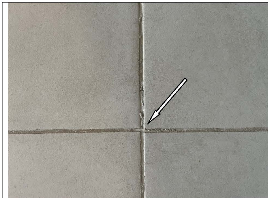
Фото №37. Дефект затирки швов напольной керамической плитки в кухне.
