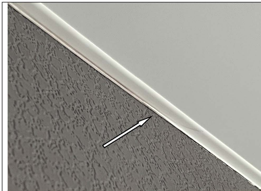
Фото №49. Дефект монтажа гибкой вставки в спальне.
