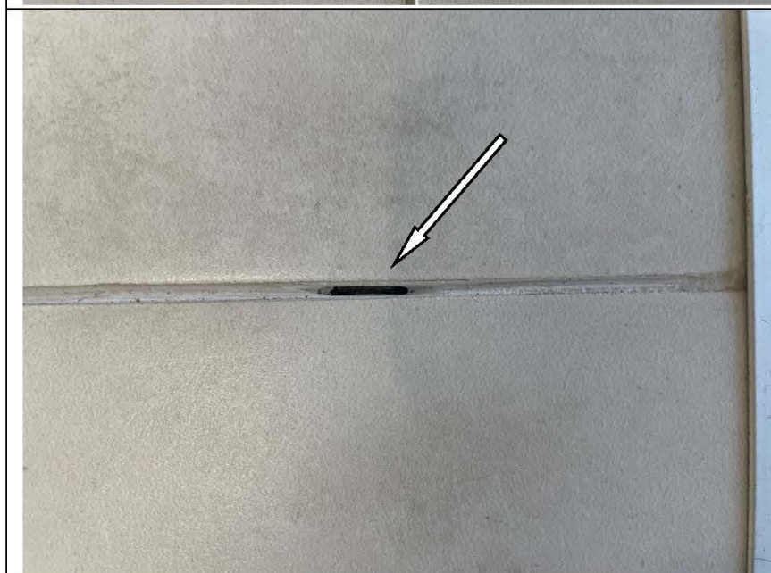
Фото №38. Дефект затирки швов напольной керамической плитки в коридоре.
